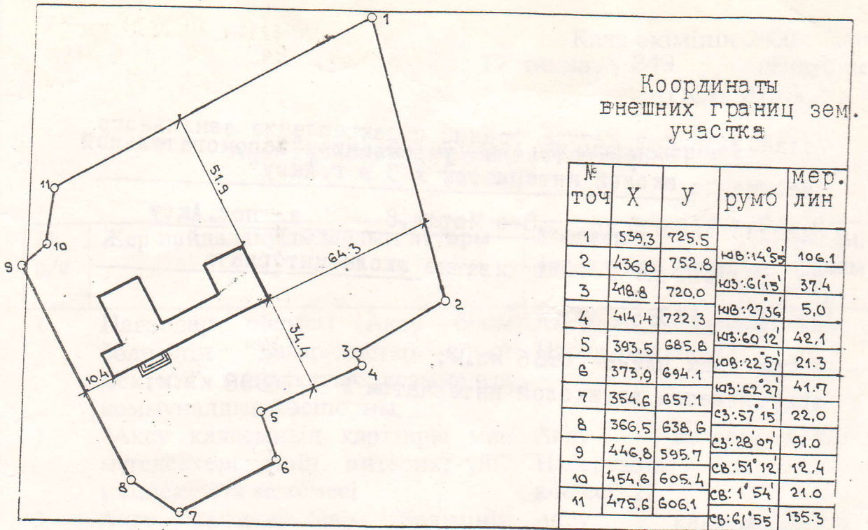
Ситуационный план размещения вспомогательной школы интерната № 3 в пос. Аксу Павлодарской обл. М-1:5000
